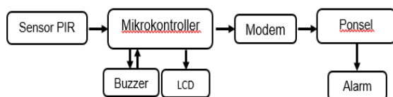
Gambar 1. Blok Diagram Rancangan (Sumber: Hasil Rancangan)
