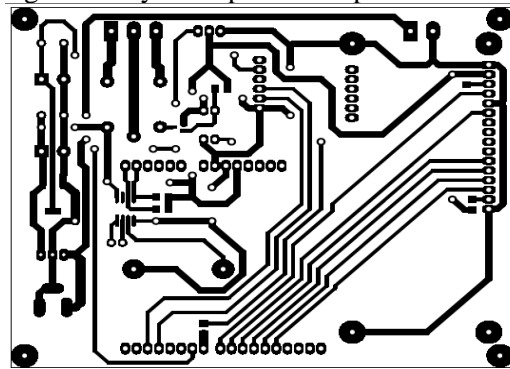
Gambar 2. Rangkaian Layout (Sumber: Hasil Rancangan)
